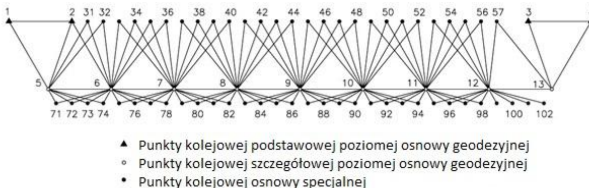
Rys. Schemat rozmieszczenia punktów kolejowej osnowy geodezyjnej
