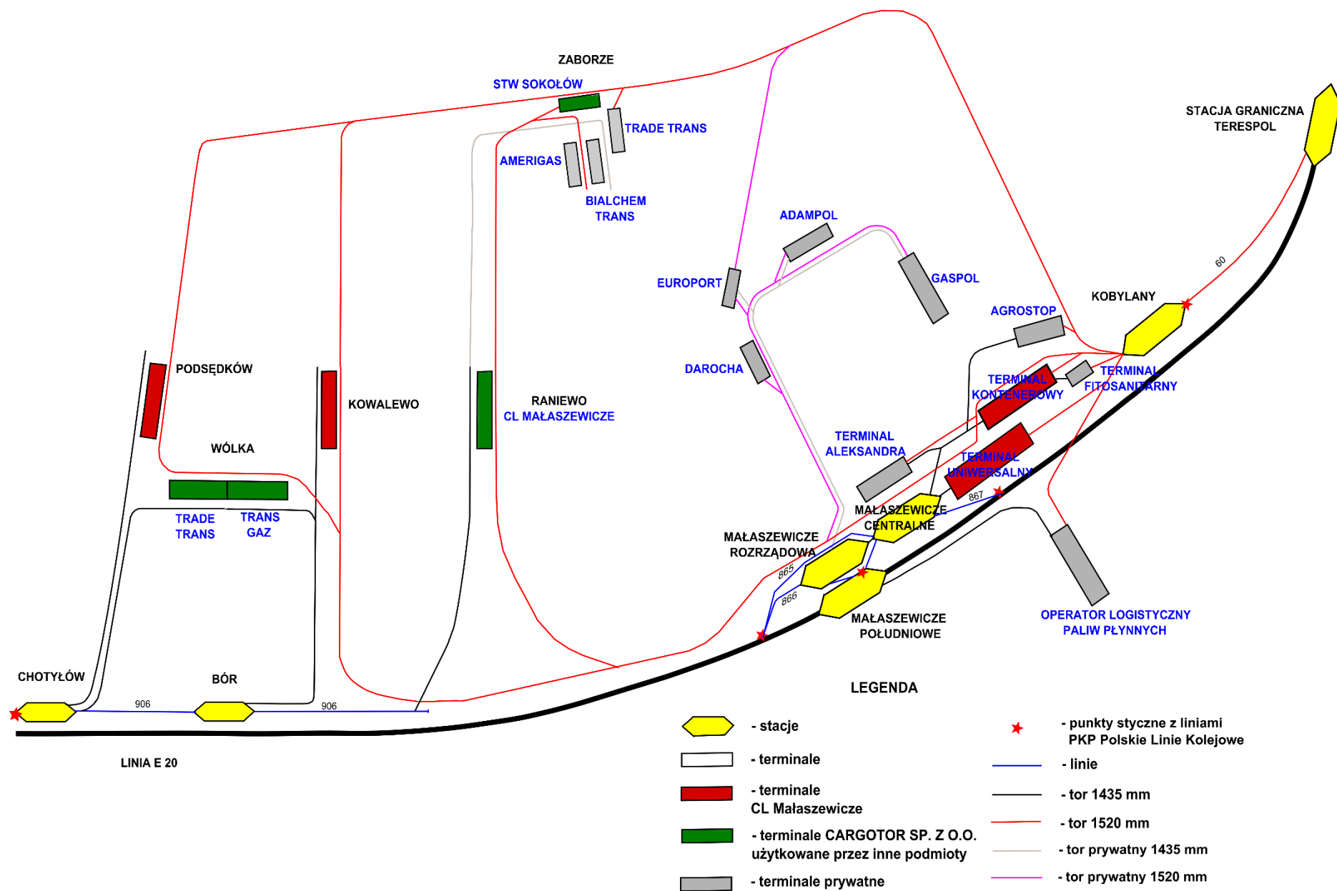
Schemat układu bocznic kolejowych w rejonie przeładunkowym Małaszewicze
